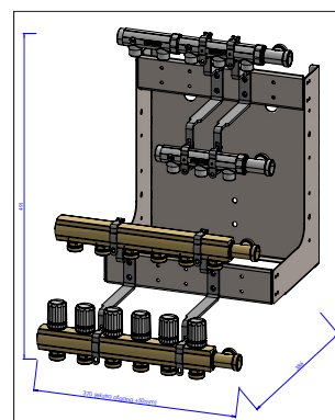
Standard SKAKTLØSNING med 6 gulvvarme-, 5 koldtvands- og 3 varmtvandskredse.
