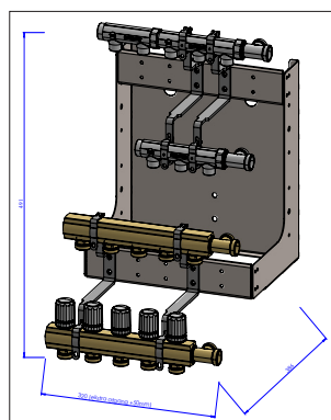
Standard SKAKTLØSNING med 5 gulvvarme-, 5 koldtvands- og 3 varmtvandskredse.
