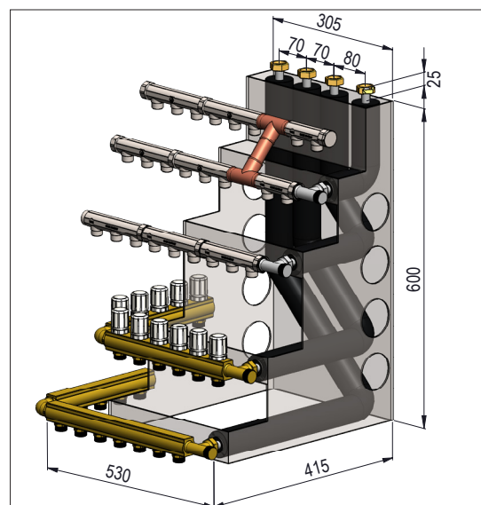
Max. bestykning af et BUNDMODUL for at det kan være i et 60 cm skab. 12 gulvvarme-, 16 koldtvands- og 9 varmtvandskredse.
